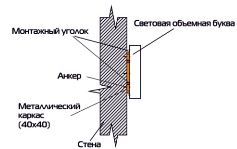
разрез А-А
